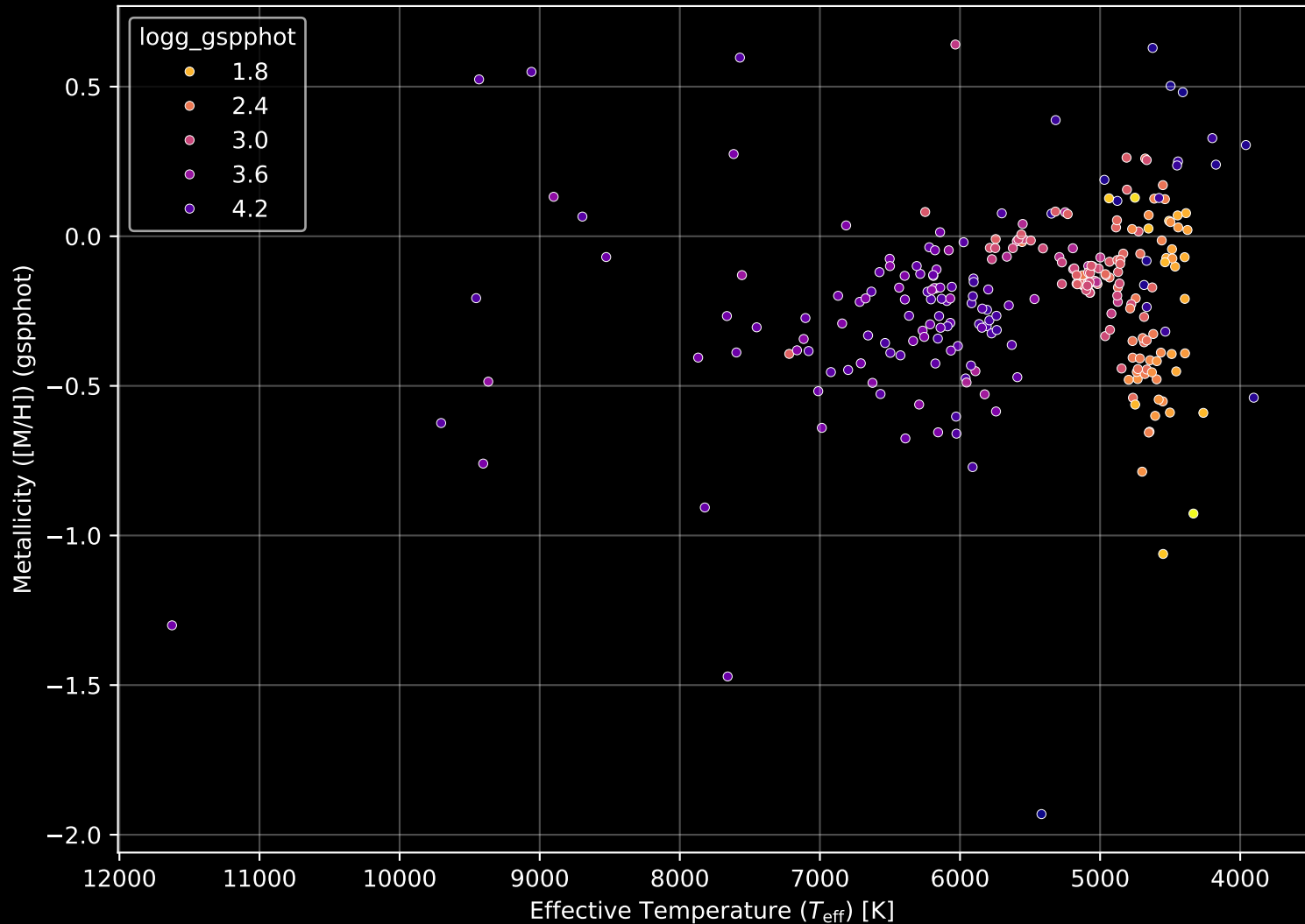
APOGEE DR17 Field: [240-12] Stellar Population Parameters (n= 265)
